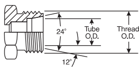
Male 24° Cone
